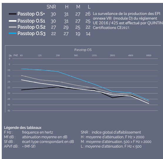
COURBES D'ATTENUATIONS
