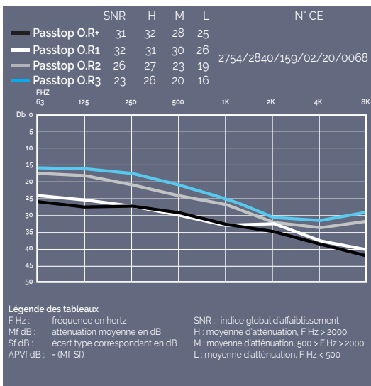
COURBES D'ATTENUATIONS
